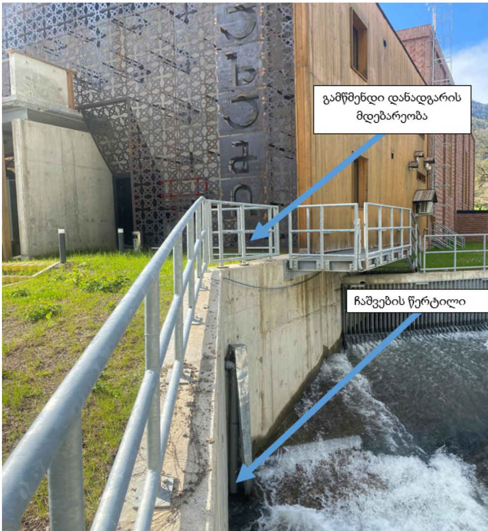
სურათი 3.5. ბიოლოგიური გამწმენდი ნაგებობის და ჩამდინარე წყლების ჩაშვების წერტილის განლაგების სქემა
