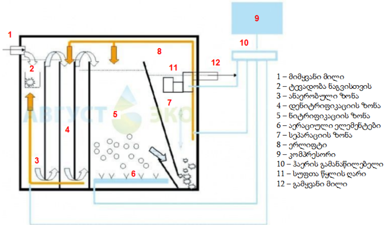
სურათი 3.2. დანადგარის სქემა
